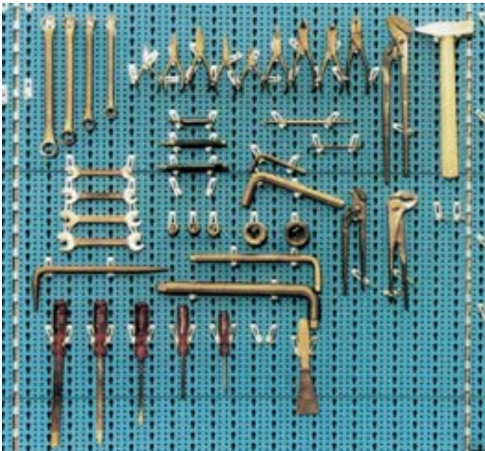
Bild 13-1: Funkenarme Werkzeuge müs- sen besonders sorgfältig, je nach dem Einsatzort, ausgewählt werden
