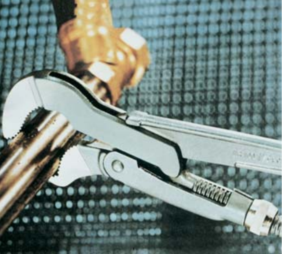
Bild 8-4: Eckrohrzange mit besonders geformtem Maul
