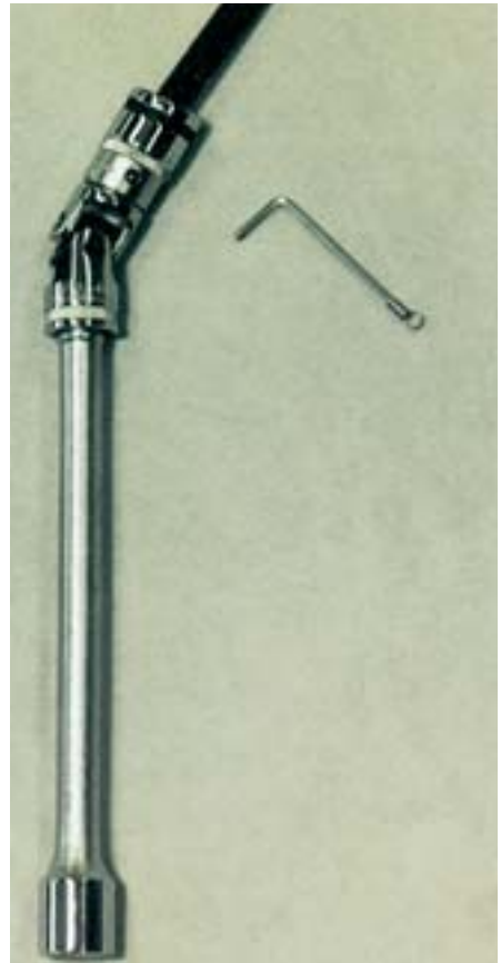
Bild 7-3: Kreuzgelenk durch nachziehbare Schraube gegen Wegkippen gehindert
