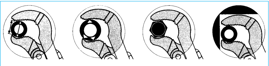
Bild 8-5: Maulform der Rohrzanze Bild 8-4 an verschiedenen Profilen
