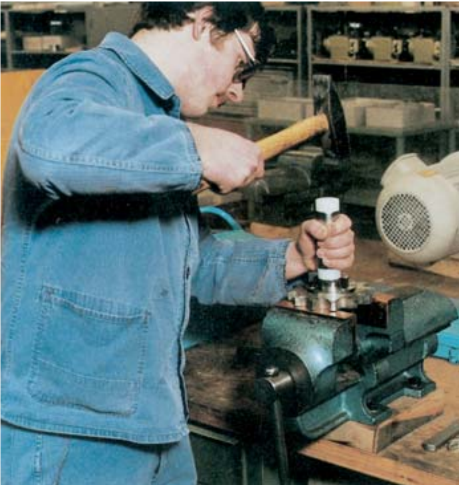
Bild 4-2: Rückschlagarm und schonend lässt sich mit diesem Dorn ein Lager treiben
