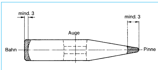
Bild 2-2: Schematischer Verlauf der Härtezonen eines Schlosserhammers
